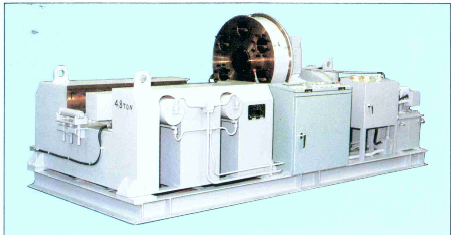
写-30 タレット付全自動パイプレデューサ(PRT-4S)
