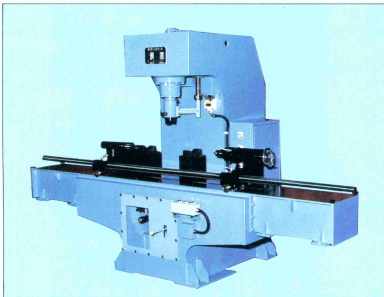
写一13 30Ton C形歪取りプレス(丸棒歪取り専用機)
