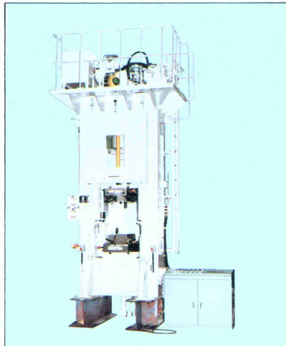
写一35 ノックアウト付200Ton門形プレス
