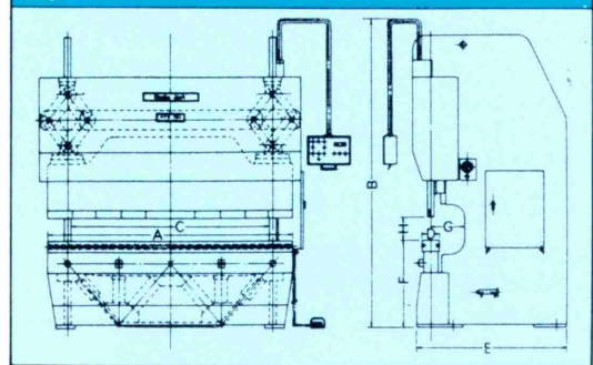
図3 100TON・150TON用
