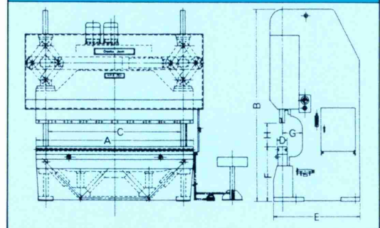
図4 200TON・250TON用
