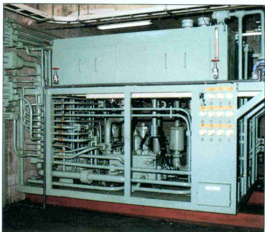
油圧ポンプユニット
