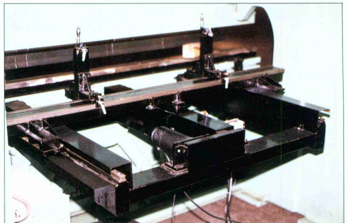
写真7 BGE形バックゲージ
