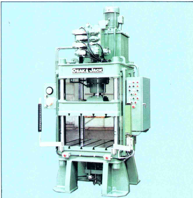
写-25 ダイクッション付100Ton 4柱式プレス (テーブル寸法800×800mmデーライト500mm)
