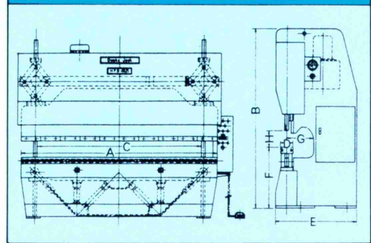
図2 50TON・75TON用
