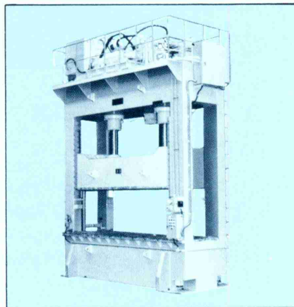
写-19 500Ton門形プレス (HPA-500)
