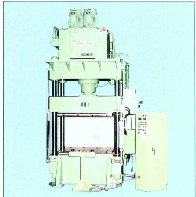
写-26 熱板付150Ton 4柱式プレス (テーブル寸法1100×900mm)
