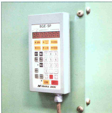
写真6 BGE形バックゲージ用コントローラー
