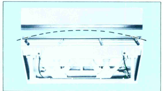
写-5 ベッド「中央撓み」補正機構(特許)
